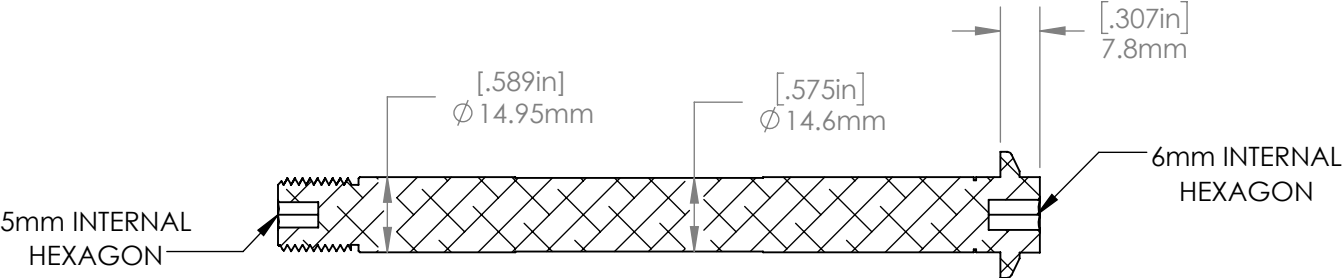
SECTION A-A SCALE 1 : 1.5
