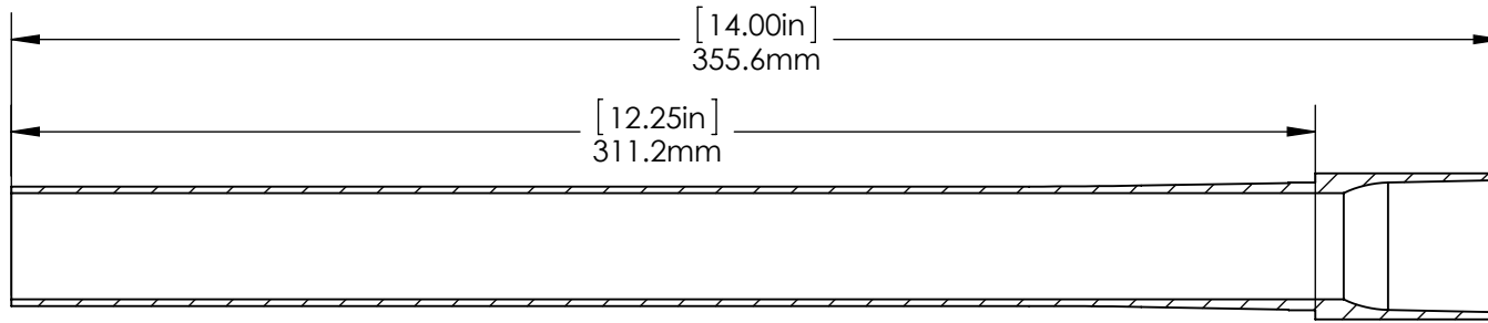
SECTION A-A SCALE 1 : 2
