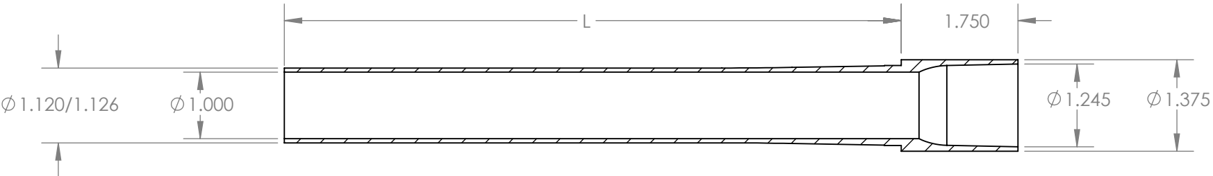
SECTION A-A SCALE 1 : 2
